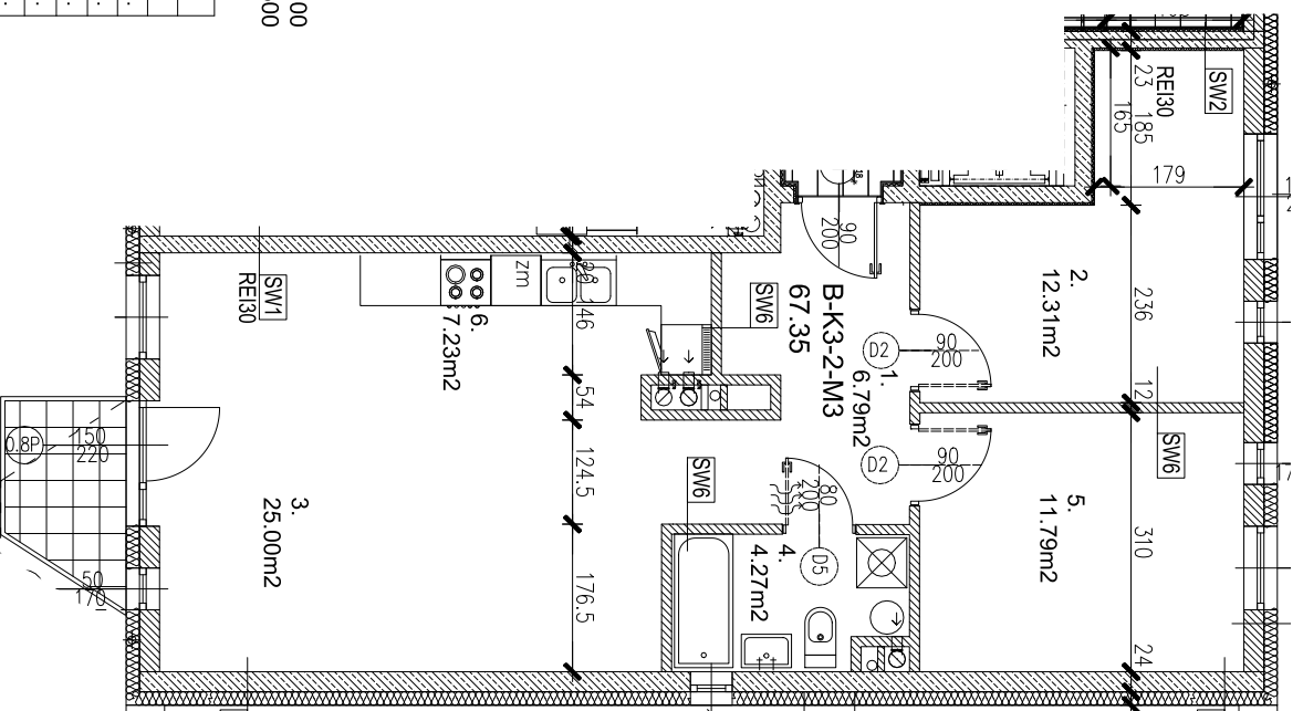
RZUT MIESZKANIA - SKALA=1:100 RZUT KONDYGNACJI +2 - SKALA=1:500
