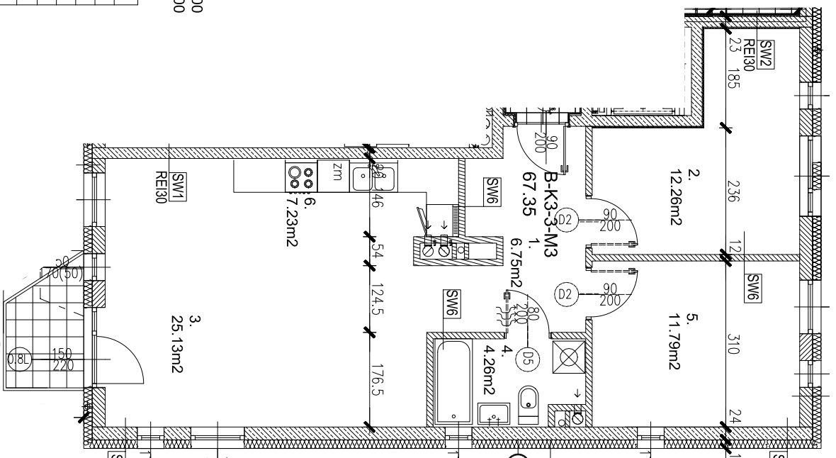
RZUT MIESZKANIA - SKALA=1:100 RZUT KONDYGNACJI +3 - SKALA=1:500
